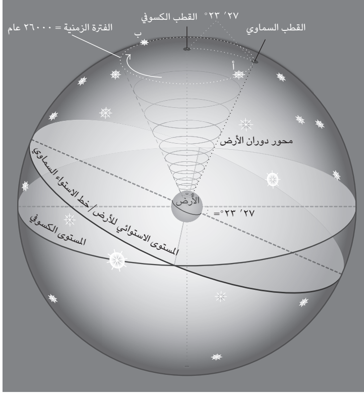
شكل ٢: المبادرة (المنظر بطلمي؛ التفسير كوبرنيكى).
