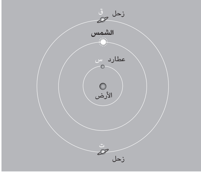
شكل ٢: الاقتران والتقابل (لو كان رأي بطليموس صحيحًا).
