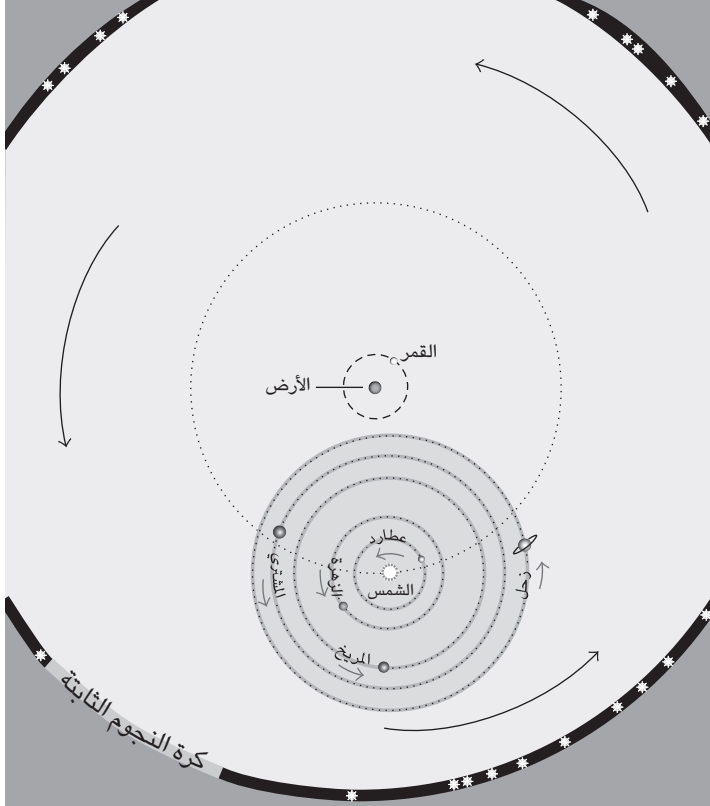
شكل ١: كون تيكو براهي (مقياس الرسم: مماثل لمقياس رسم كوبرنيكوس).
