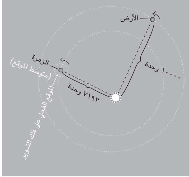
شكل ٦: المدار الزُّهري حسب رأي كوبرنيكوس.
