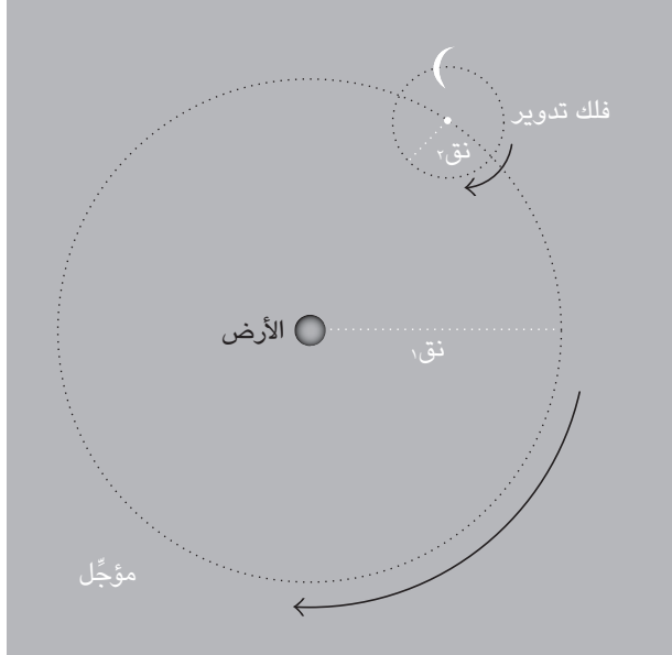
شكل ٦: فلك التدوير (حسب الرأي البطلمي والكوبرنيكي).
