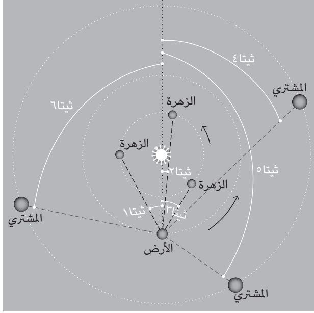
شكل ٣: الاستطالة الزاوية (حسب رأي كوبرنيكوس).
