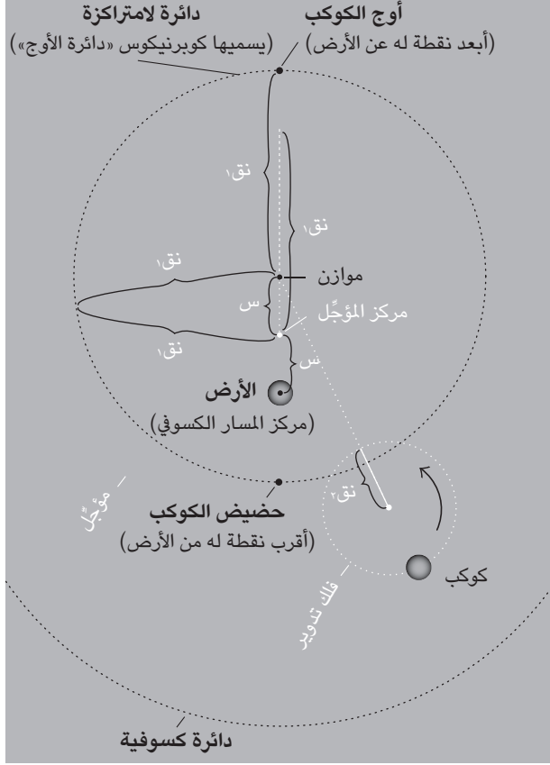
شكل ٧: الموازن (حسب رأي بطليموس فقط).
