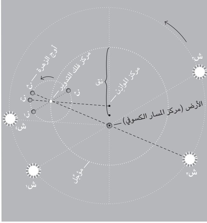
شكل ٥: المدار الزُّهري حسب رأي بطليموس.
